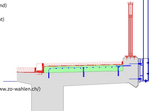
Im Querschnitt: So sehen die Träger (blau) nach dem Entfernen der Schilder aus (Grafik PD Baudirektion)
